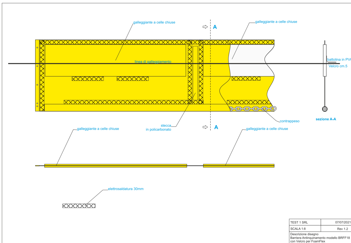
Sezione A-A - Barriera Antinquinamento modello BRFF18 con Velcro per FoamFlex (TEST1 SRL, Rev 1.2, 07/07/2021)
